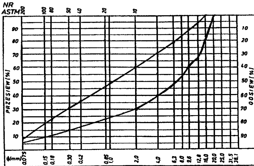
Rys. 1. Krzywe graniczne uziarnienia mieszanki mineralnej 0+20 mm do warstwy scieralnej z betonu asfaltowego dla KR 1-2
