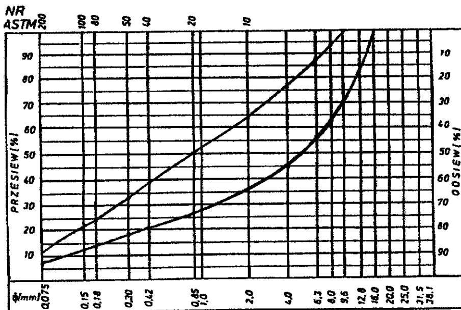
Rys. 2. Krzywe graniczne uziarnienia mieszanki mineralnej 0+16, 0+12,8 mm do warstwy scieralnej z betonu asfaltowego dla KR 1-2
