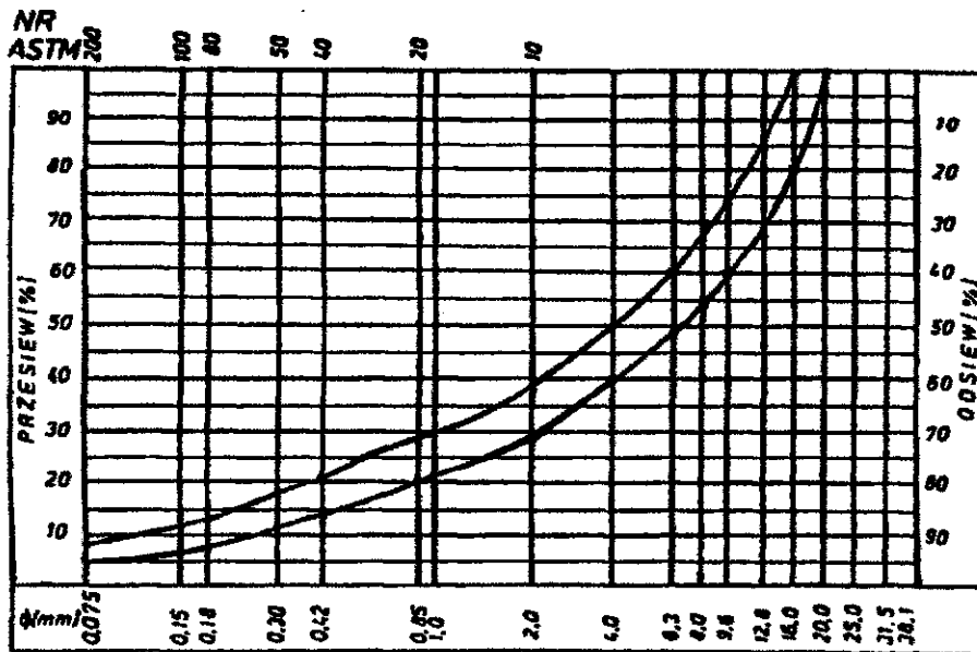
Rys. 4. Krzywe graniczne uziarnienia mieszanki mineralnej 0+20 mm do warstwy ściaralnej z betonu asfaltowego dla KR 3-6
