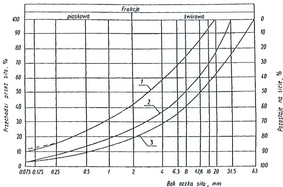
Rysunek 1. Pole dobrego uziarnienia kruszyw przeznaczonych na podbudowy i nawierzchni wykonywane metodą stabilizacji mechanicznej
