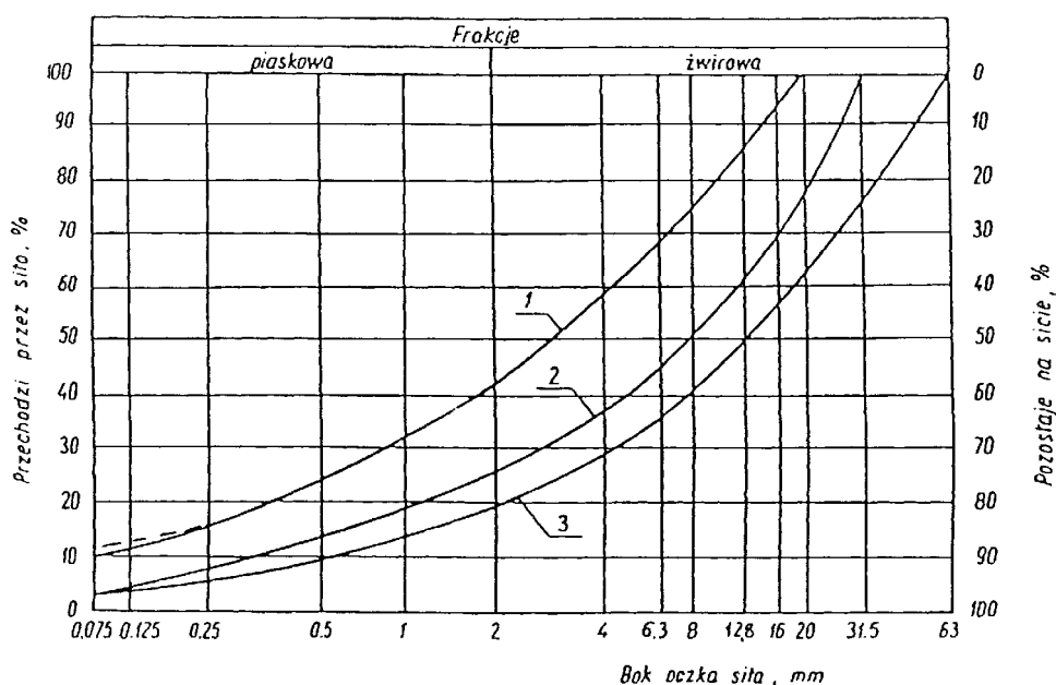
Rysunek 1. Pole dobrego uziarnienia kruszywa przeznaczonych na podbudowy i nawierzchni wykonywane metodą stabilizacji mechanicznej
