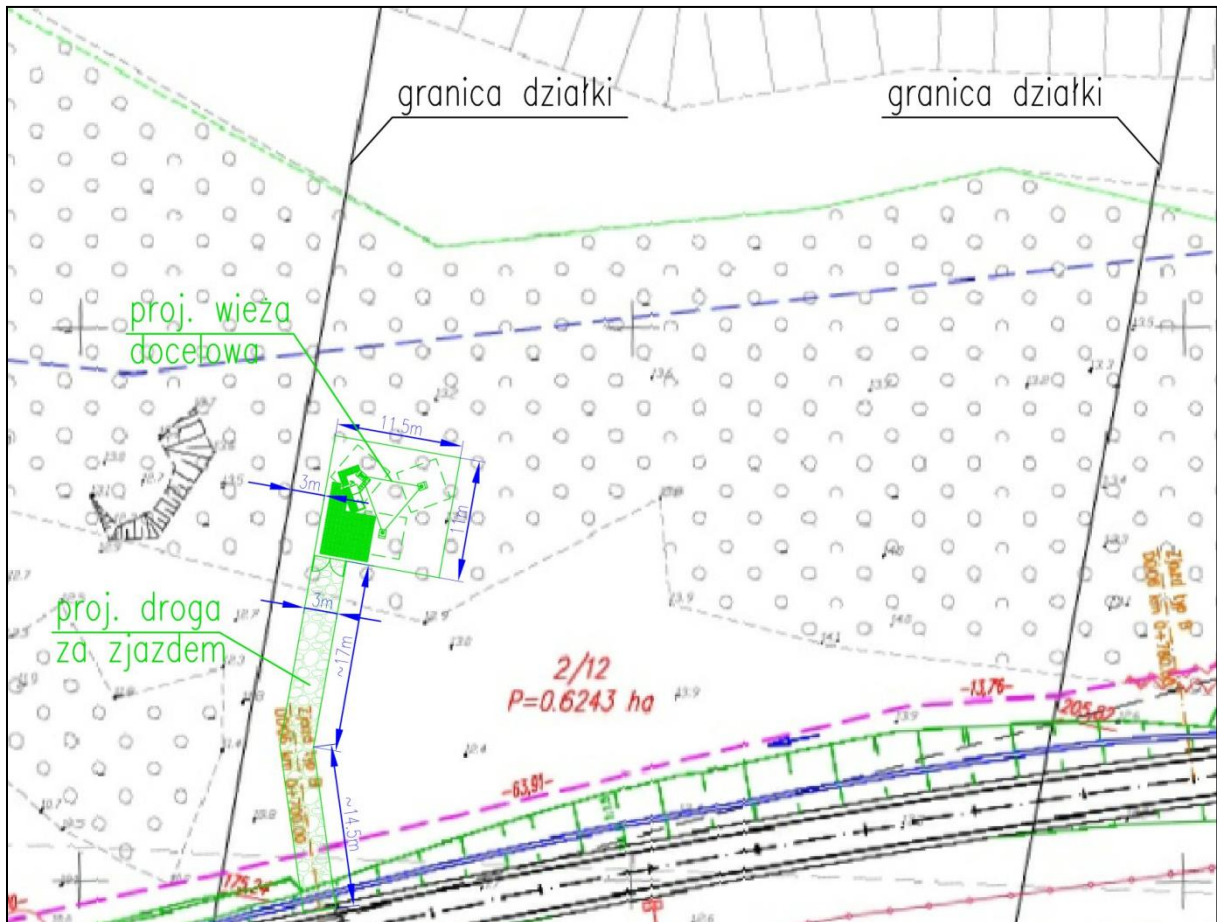
Projekt zagospodarowania terenu
